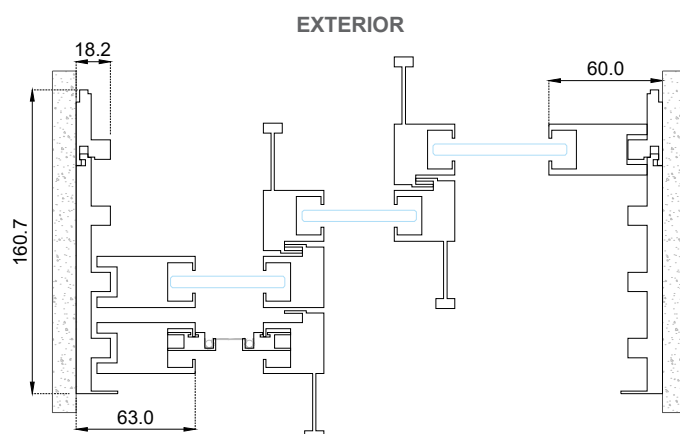
Sección A-A'
