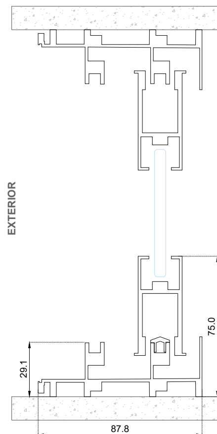
Sección B-B'
