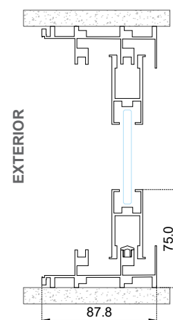
Sección B-B'
