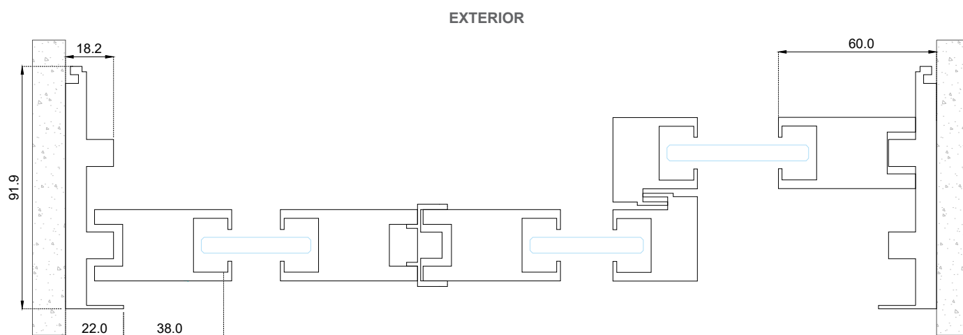
Sección A-A'
