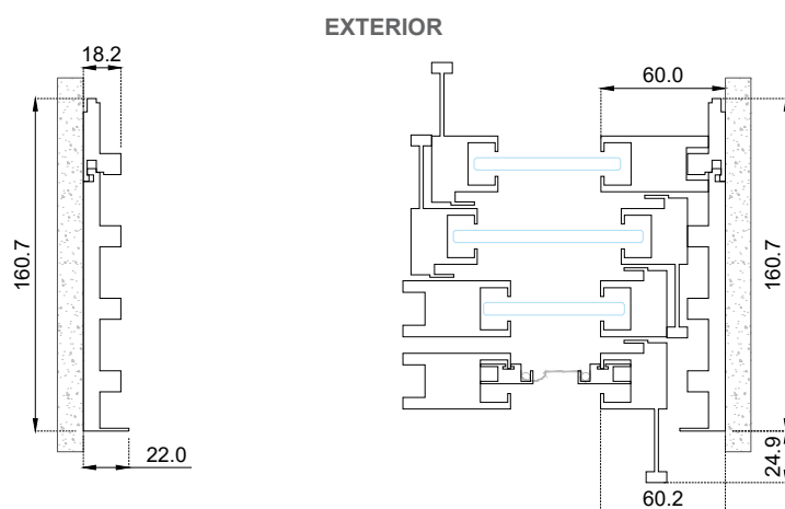
Sección A-A'
