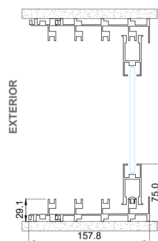
Sección B-B'
