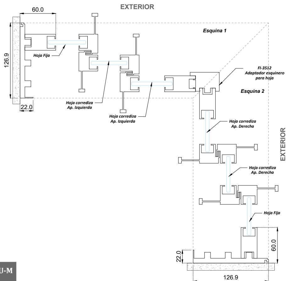
Corrediza por interior Sección A-A'
