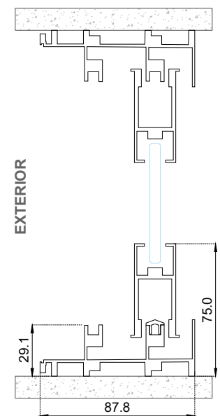
Sección B-B'
