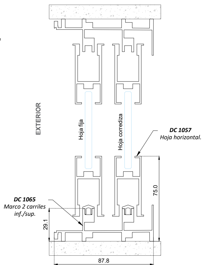
Sección B-B'
