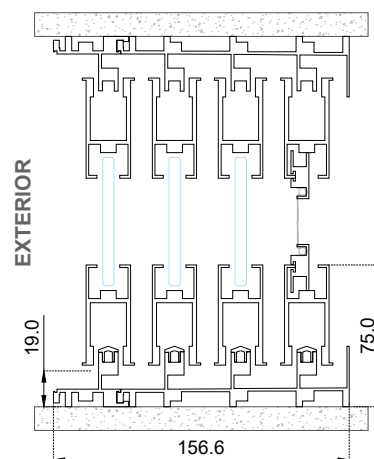
Sección B-B'
