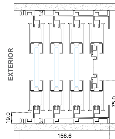
Sección B-B'
