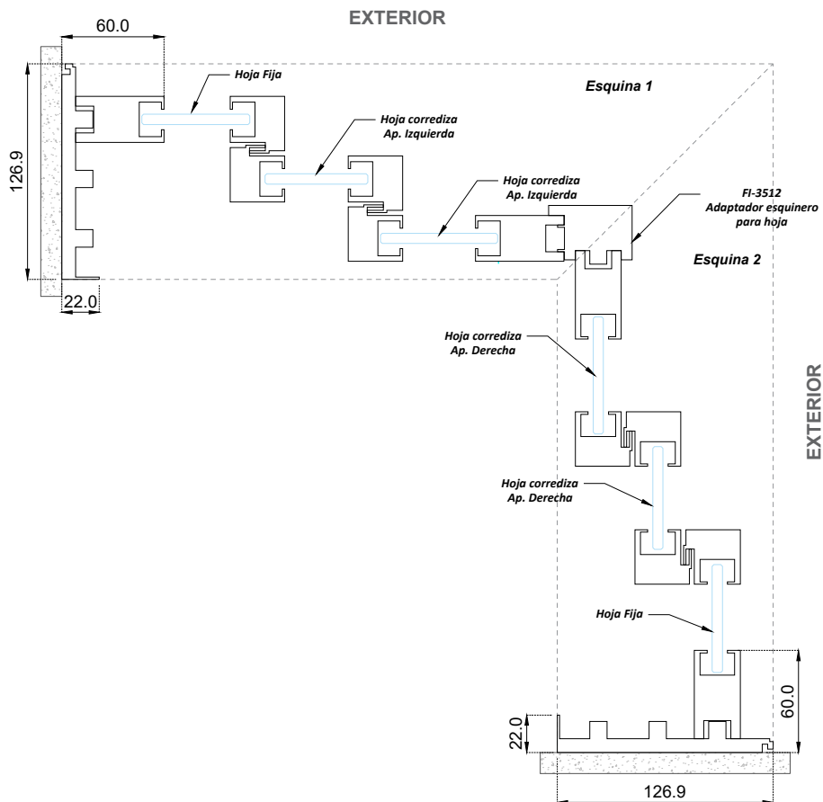
Corrediza por interior Sección A-A'
