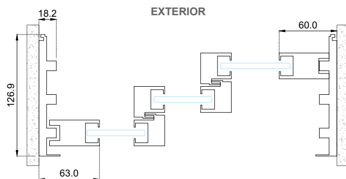
Sección A-A'
