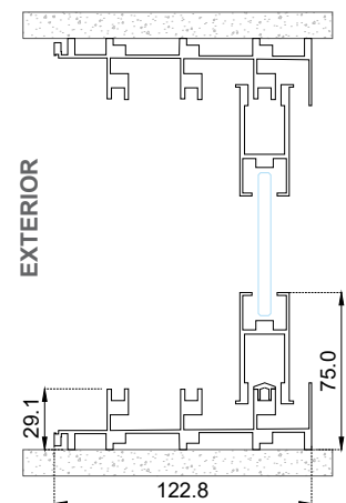
Sección B-B'
