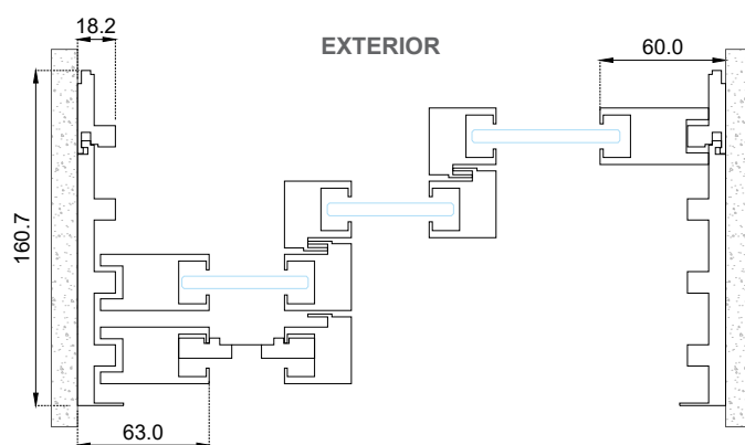
Sección A-A'
