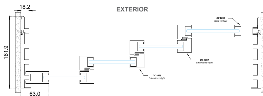
Sección A-A'
