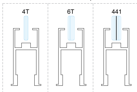
Detalle de espesor de vidrio
