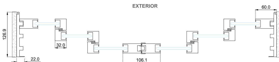
Sección A-A'
