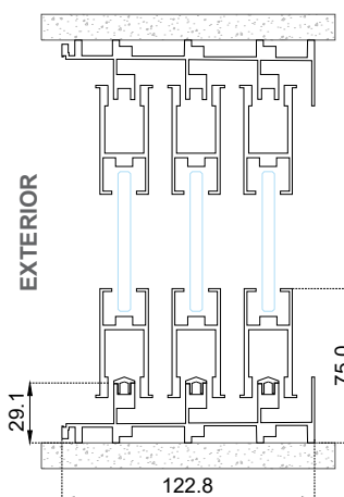
Sección B-B'
