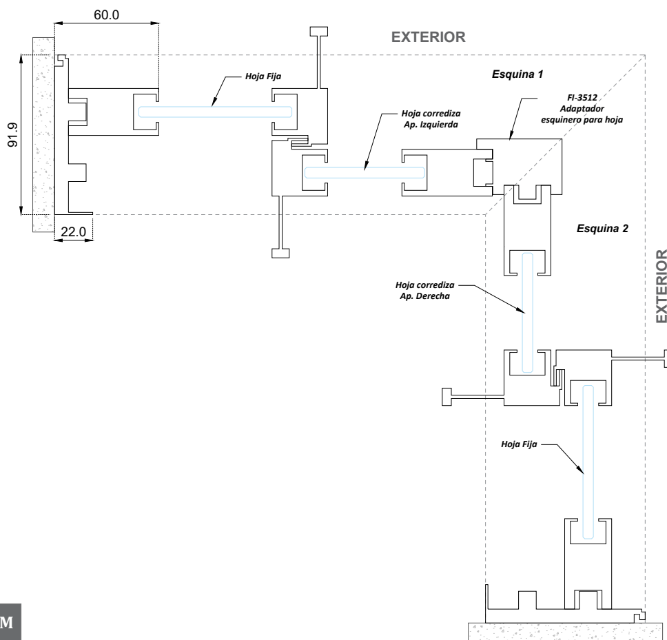
Corrediza por interior Sección A-A'
