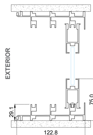
Sección B-B'
