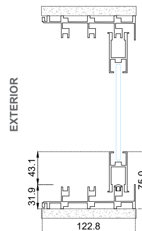
Sección B-B'
