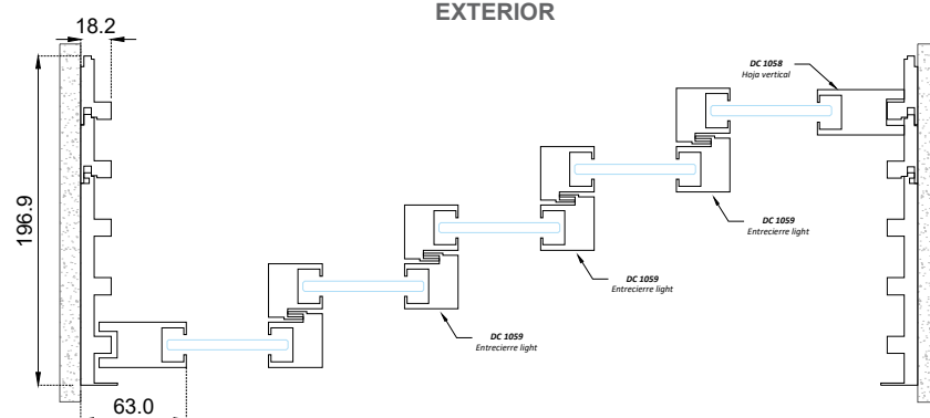
Sección A-A'
