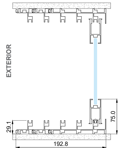
Sección B-B'
