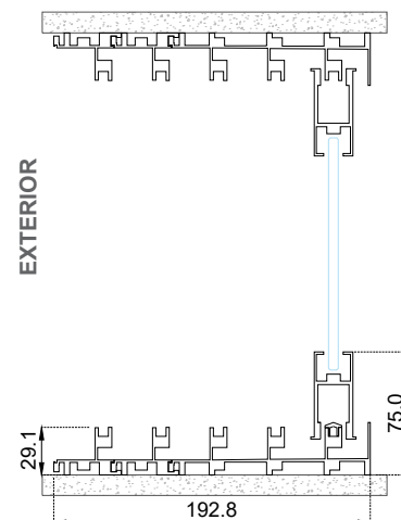
Sección B-B'
