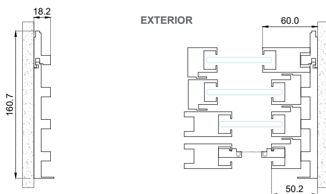
Sección A-A'
