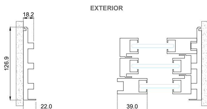
Sección A-A'
