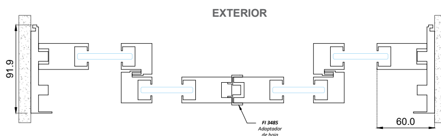
Sección A-A'
