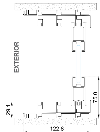
Sección B-B'
