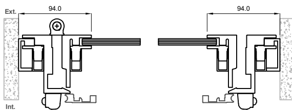
Sección C-C'
