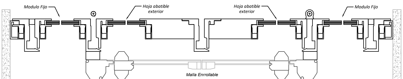
Sección E-E'
