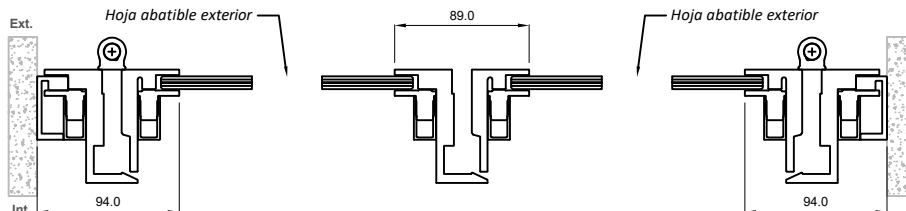
Abatible apertura exterior Sección B-B'
