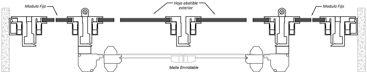
Sección D-D'
