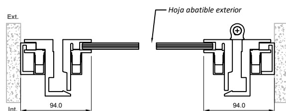
Abatible apertura exterior Sección B-B'
