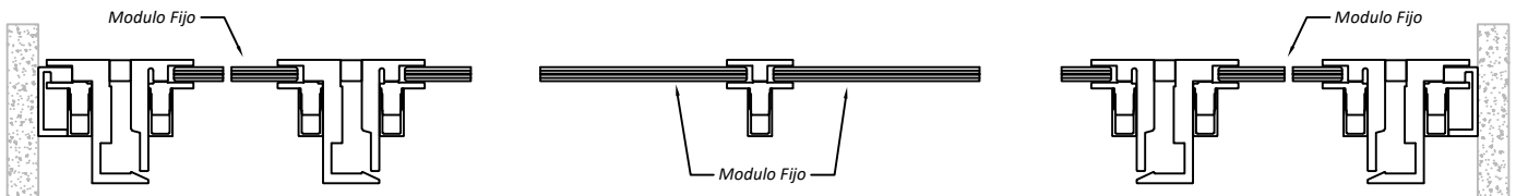
Sección C-C'
