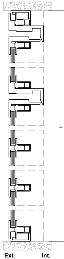
Fijos laterales con Puerta apertura exterior Sección A-A'
