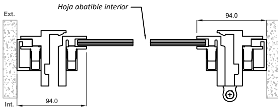
Abatible apertura interior Sección B-B'
