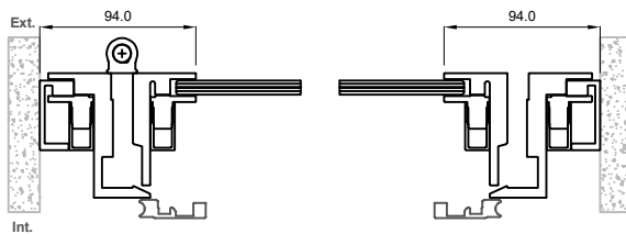
Sección C-C'
