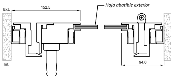
Sección C-C'
