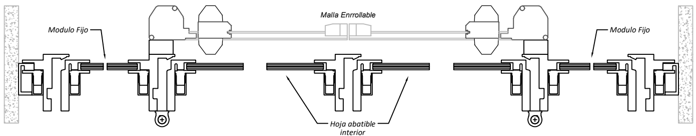
Sección E-E'
