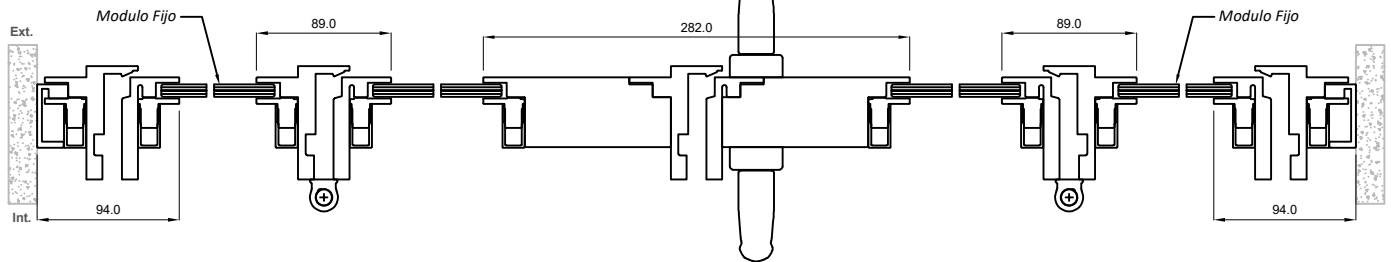
Abatible apertura interior Sección E-E'
