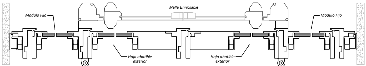
Sección E-E'
