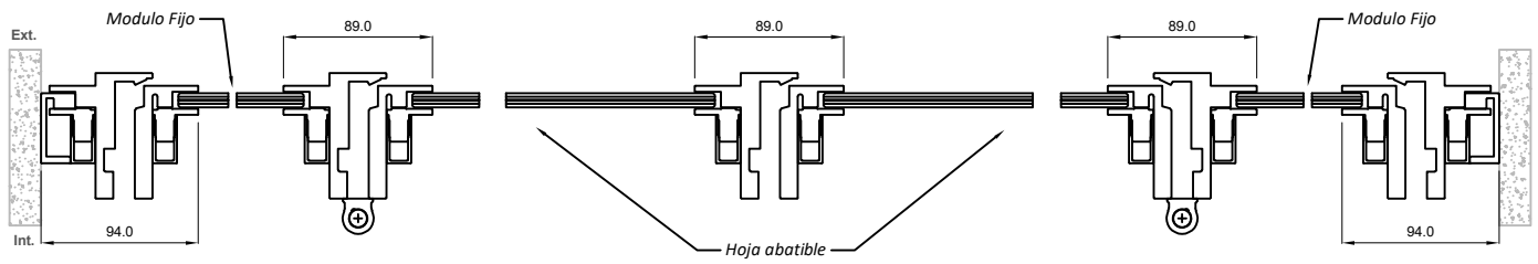
Abatible apertura interior Sección D-D'
