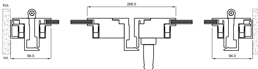
Sección C-C'
