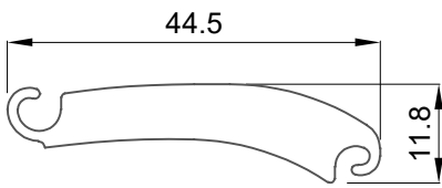
FI-2742 LAMA CIEGA
