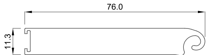
313029 REMATE/TERMINAL PEQUEÑO
