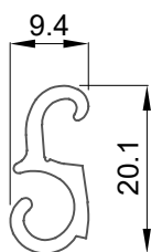
FI-5593 VARILLA DE UNIÓN
