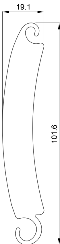
FI-5591 LAMA CIEGA
