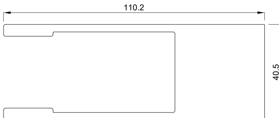
FI-4230 GUIA LATERAL
