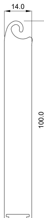
313031 REMATE/TERMINAL PEQUEÑO
