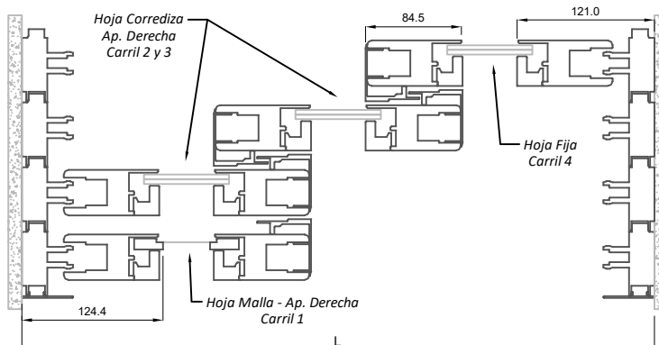
Sección A-A'
