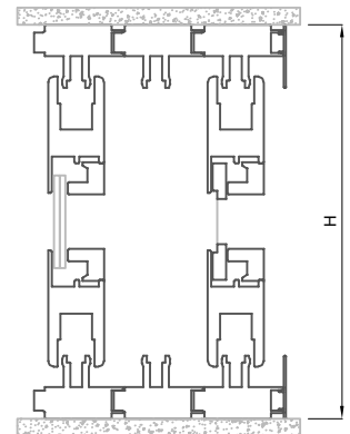
Corrediza por exterior Sección B-B'
