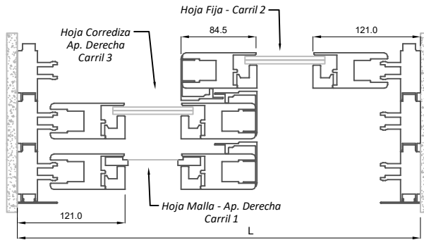
Corrediza por interior Sección A-A'
