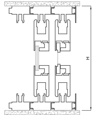
Corrediza por interior Sección B-B'
