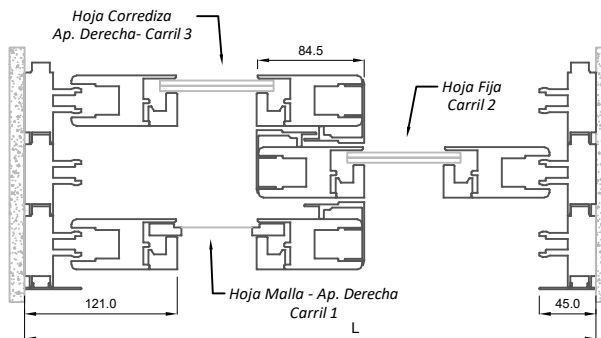
Corrediza por exterior Sección A-A'
