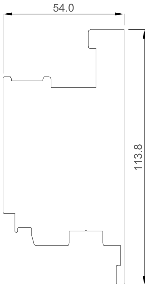
FI-4864 HOJA ABATIBLE APERTURA EXTERIOR
