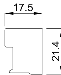
FI-4261 JUNQUILLO RECTO
