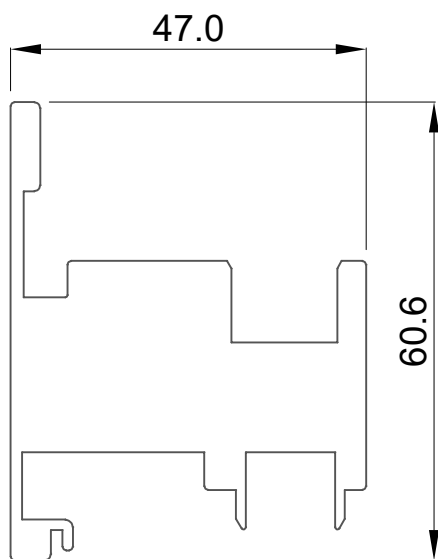
FI-4862 INVERSOR DE HOJA
