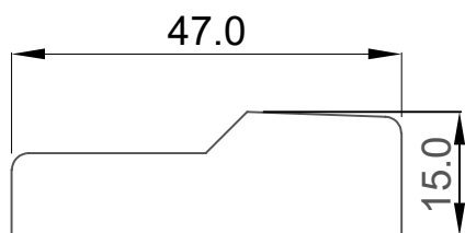
FI-4866 SARDINEL APERTURA EXTERIOR
