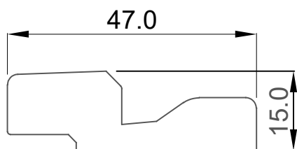
FI-5111 SARDINEL APERTURA INTERIOR
