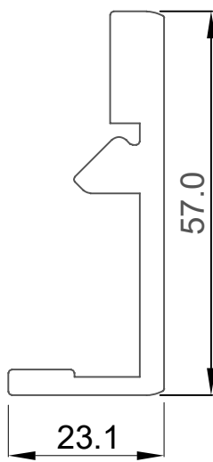
FI-4868 BATIENTE ZOCALO
