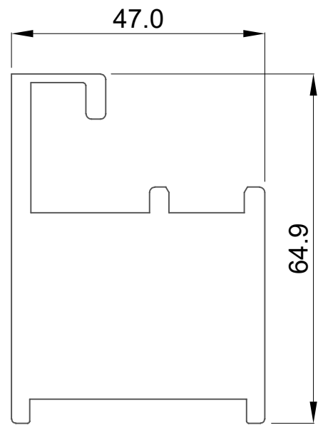
FI-4263 MARCO PARA FIJO
