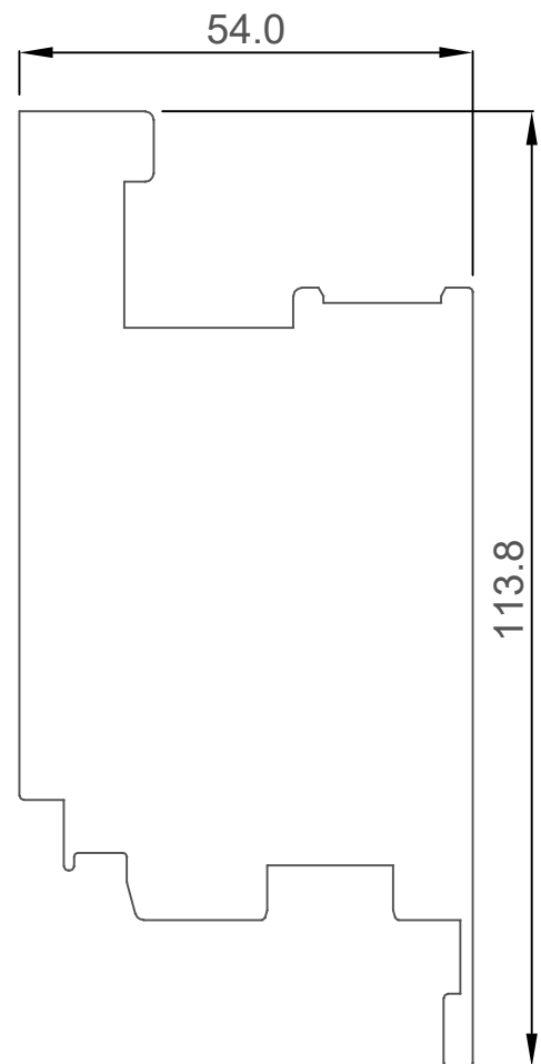
FI-4861 HOJA ABATIBLE APERTURA INTERIOR
