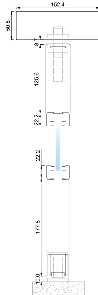
Corte Vertical Sección B-B'
