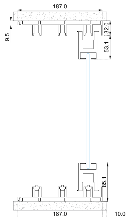
Sección B-B'
