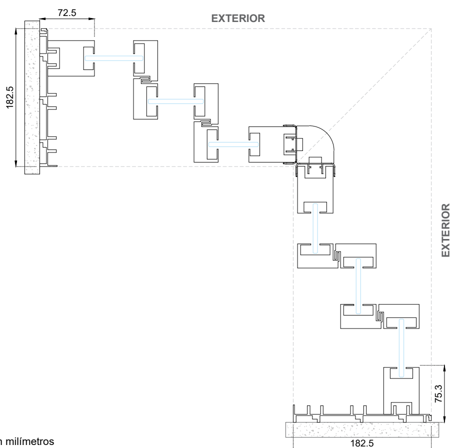
Sección A-A'
