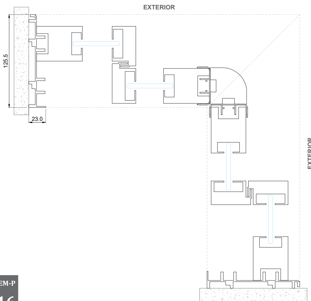
Sección A-A'
