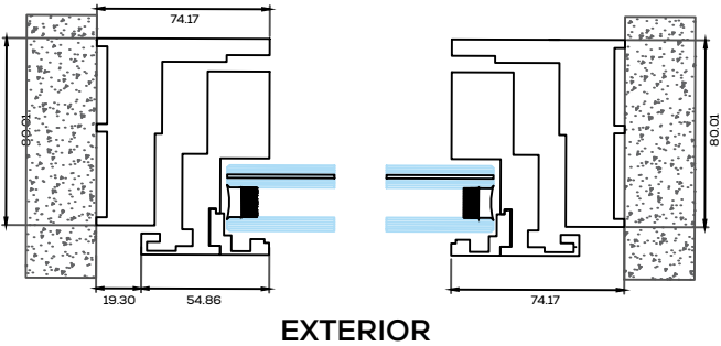
Corte Horizontal
