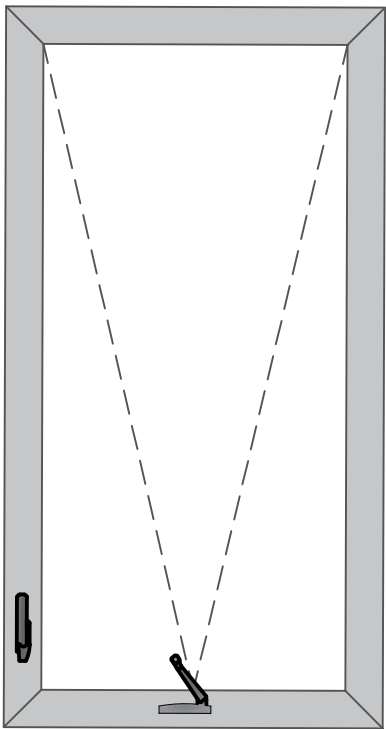
Ventana proyectable
